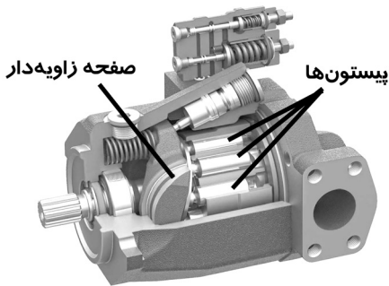
پمپ پیستونی با صفحه زاویه دار
