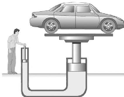
پاورونیت هیدرولیک
