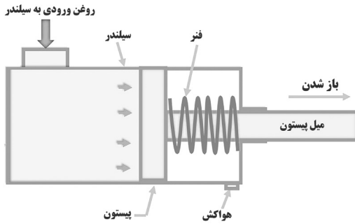
سیلندر هیدرولیک یک‌کاره (کورس رفت)
