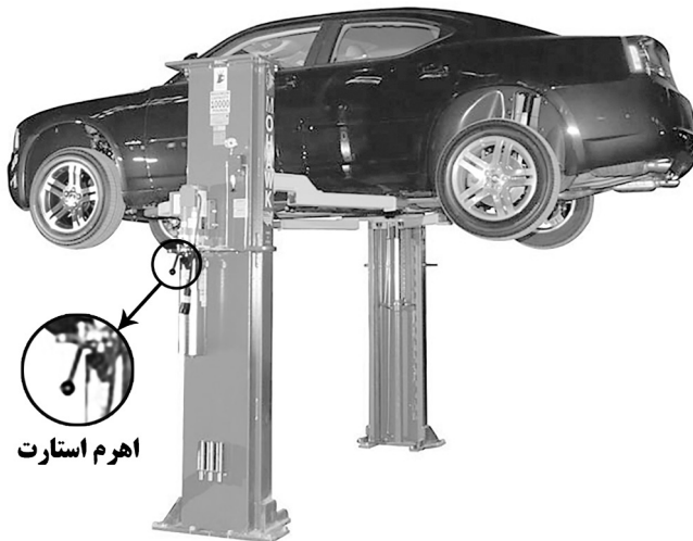
جک هیدرولیک بالابر خودرو
