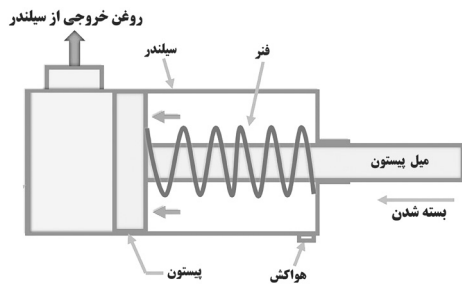
سیلندر هیدرولیک یک‌کاره (کورس برگشت)
