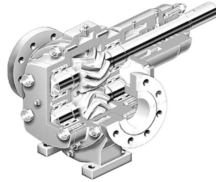
پمپ دنده جناعی (Herringbone Gear Pump)
