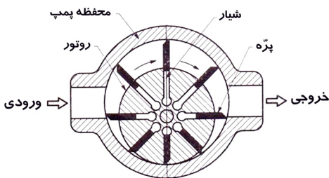
پمپ پره‌ای نامتعادل
