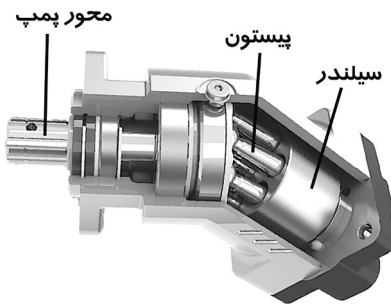
پمپ هیدرولیک پیستونی با محور خمیده
